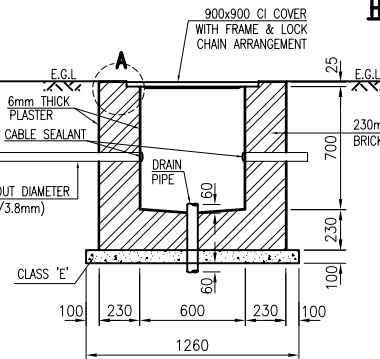
OP SECTION B-B SCALE= 1:2
